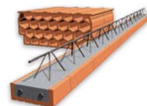
POROTHERM nosník POT + vložka MIAKO
